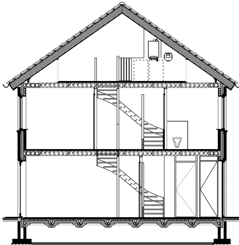
doorsnede 1:100
