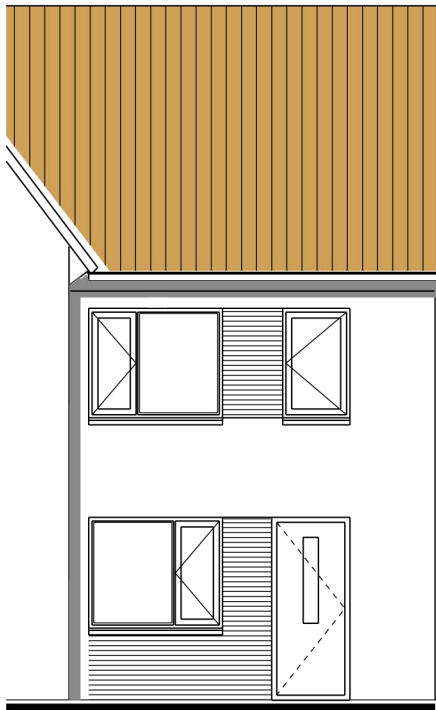
aanzicht voorgevel 1:100
